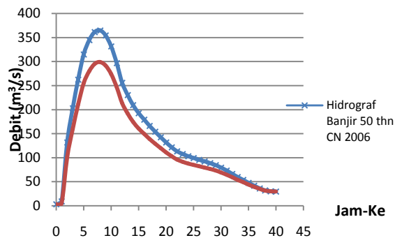
Gambar 6. Hidrograf Banjir rancangan DAS Jlantah kala ulang 50 tahun CN 2006 dan CN 2025.
