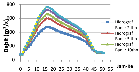
Gambar 3. Hidrograf Banjir DAS Dengkeng dari CN 2006.
