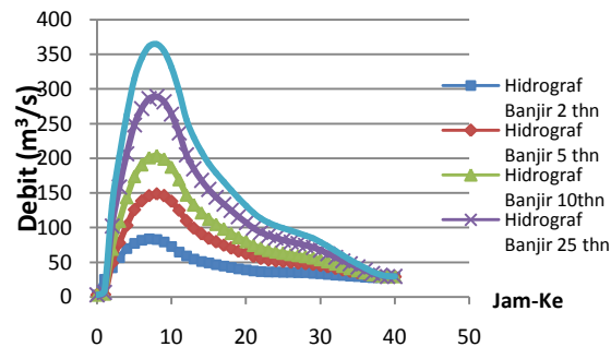
Gambar 4. Hidrograf Banjir DAS Jlantah dari CN 2006.
