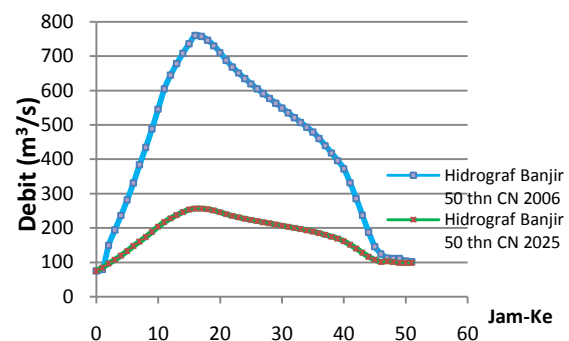
Gambar 5. Hidrograf Banjir rancangan DAS Dengkeng kala ulang 50 tahun CN 2006 dan CN 2025.
